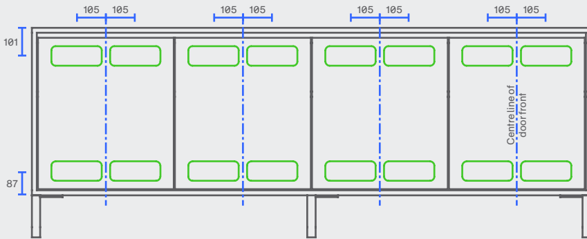
AV Cut-outs in Rear Panel. Front View
