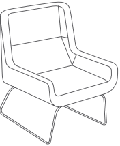
NOHUN112 Hush Low 座椅 雪橇底座 mm W 720 D 760 H 880 座 430 inch W 28.5 D 30 H 34.5 座 17
