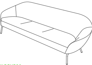
NOEVE30 Ever 三座沙发 mm W2325 D800 H760 座410 inch W91.5 D31.5 H30 座16
