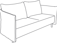
NOCLN430 Cloud Plain 2座沙发 配有低靠背 mm W1600 D750 H650 座400 inchW63 D29.5 H25.5 座15.5
