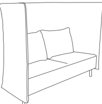
NOCLN530 Cloud Plain 2座沙发 配有高靠背 mm W1600 D750 H1300 座400 inchW63 D29.5 H51 座15.5
